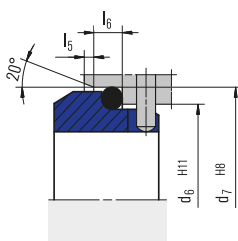
G9 (EN 12756)
