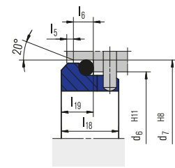
G16 (EN 12756)
