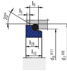
G6 (EN 12756)
